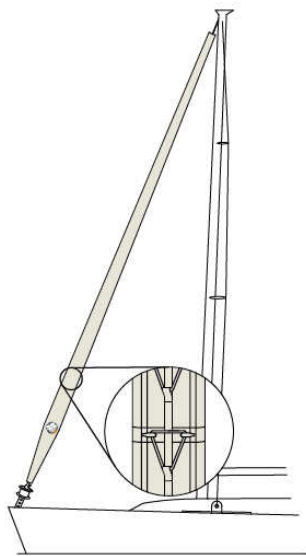
FOURREAU DE GÉNOIS
